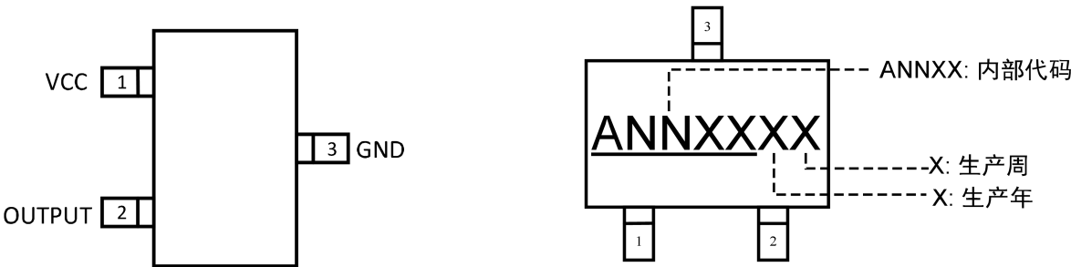
SOT23
